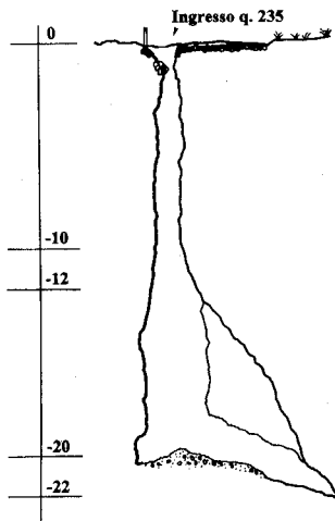
Sezione longitudinale
